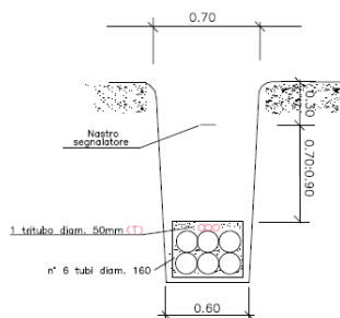
Sezione tipo di attraversamento
