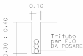
PARTICOLARE SCAVO IN MINITRINCEA IN BANCHINA ASFALTATA
