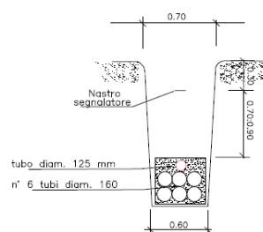
Sezione tipo di attraversamento
