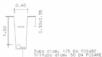
PARTICOLARE SCAVO IN ATTRAVERSAMENTO
