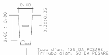
PARTICOLARE SCAVO IN CARREGGIATA/MARCIAPIEDE
