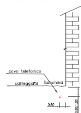
Sezione scavo su banchina
