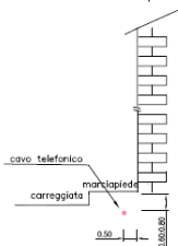
Sezione scavo su marciapiede
